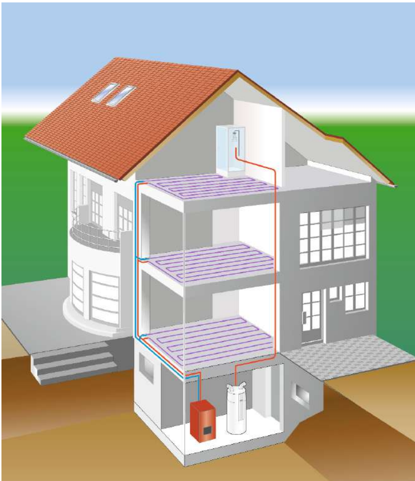
Trinkwasser-Wärmepumpe
